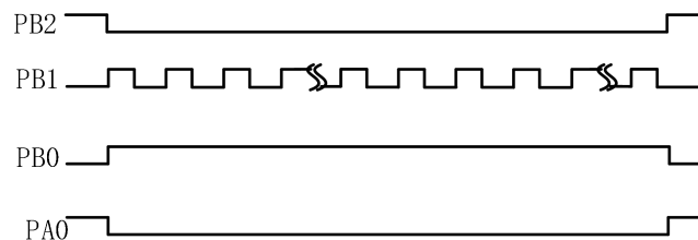
全桥 PWM 输出示例 b
